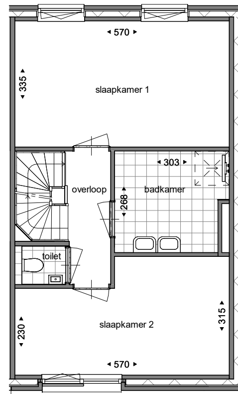
eerste verdieping
