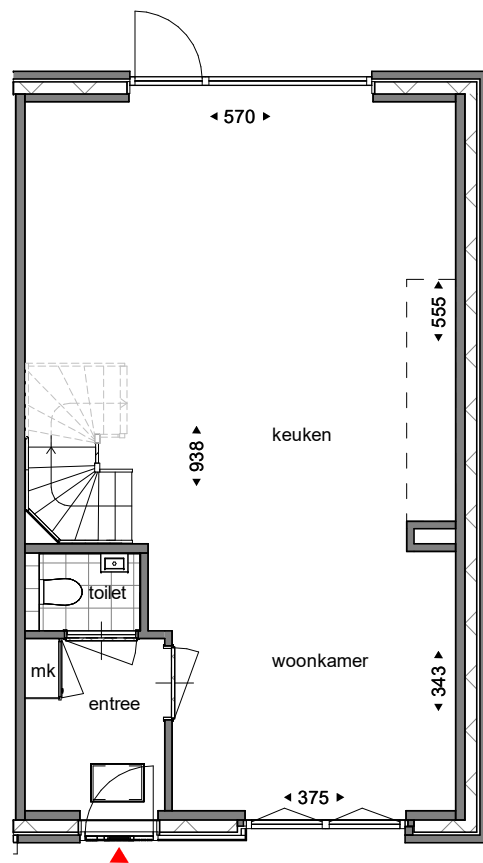
begane grond
